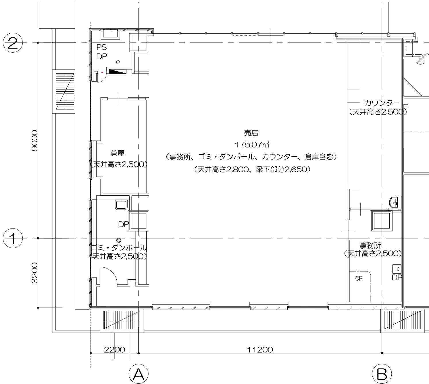
売店 平面図
